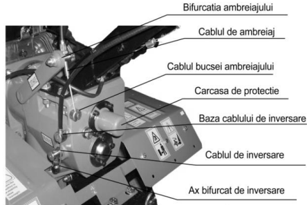
Fig. 6 – Instalarea și reglarea manetei de ambreia
